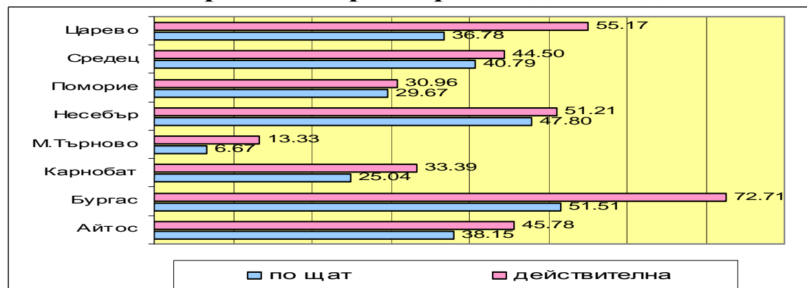
Сравнение на натовареността по щат и действителната натовареност спрямо разглежданите дела :
